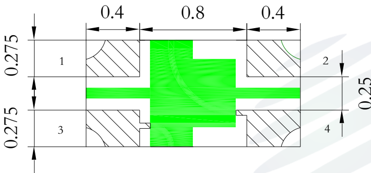
Fig.1-3 Bottom view 背面视图
