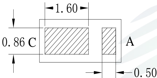
Fig. 1-3 BottomView背面视图
