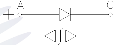
Fig. 1-4 Polarity极性
