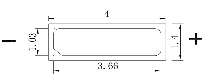
Fig.1-1 Top view 正面视图
