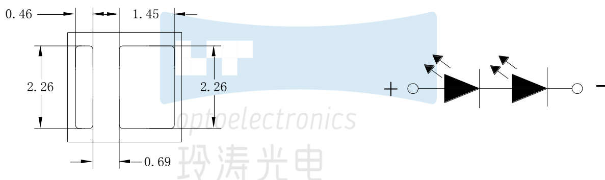
Fig.1-3 Bottom view 背面视图
