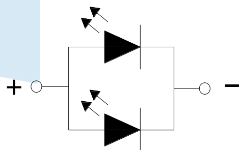
Fig.1-4 Polarity 极性
