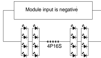
Fig.2-2ED Module connection 模組電性圖
