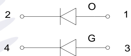
Fig.1-4 Polarity 极性
